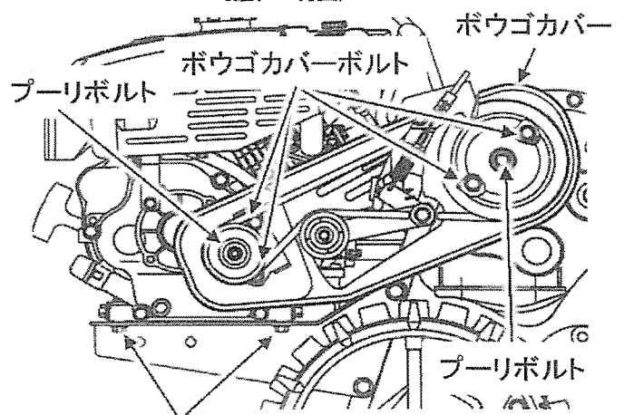
エンジン固定ボルト(4本)
