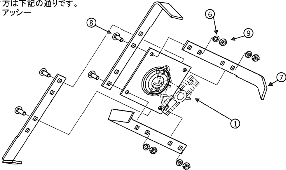
図1.ホリトリツメの取付け方 四角いツメトリツケイタを挟み込むように組付けます。
