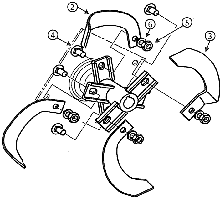
図2.コウウンツメの取付け方(1)
