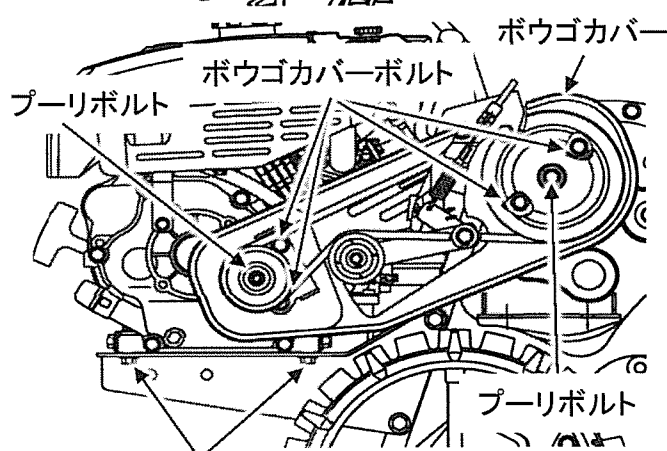
エンジン固定ボルト(4本)
