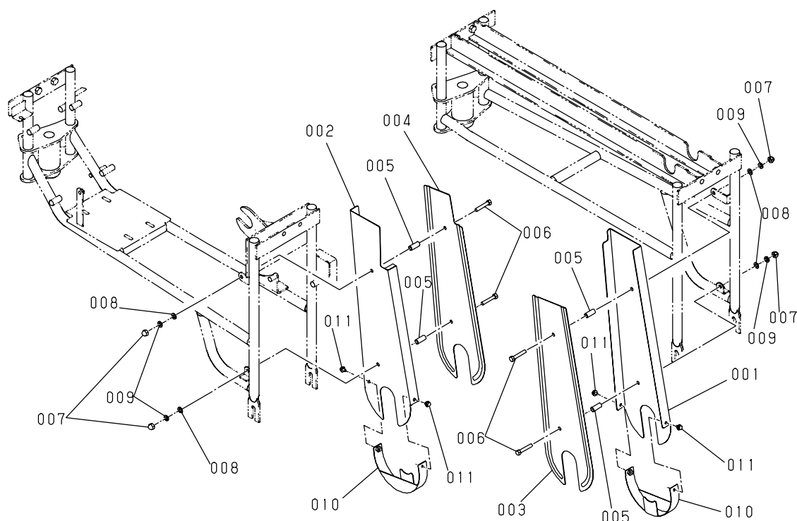
KYU-S-3 野菜運搬車
