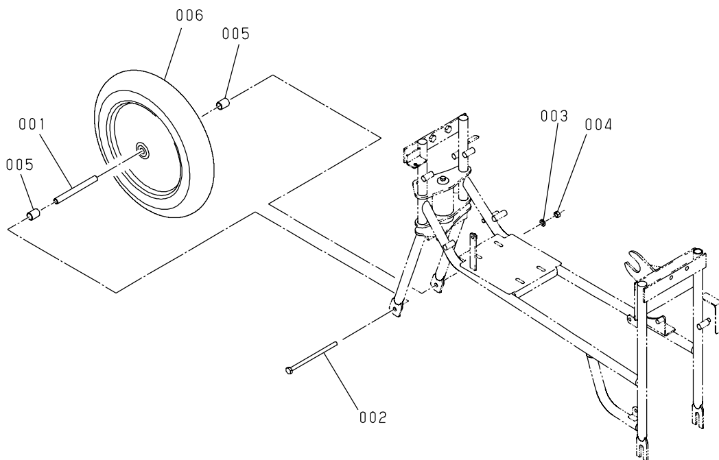
KYU-S-3 野菜運搬車
