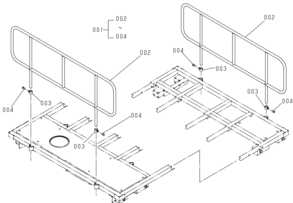
KYU-S-3 野菜運搬車
