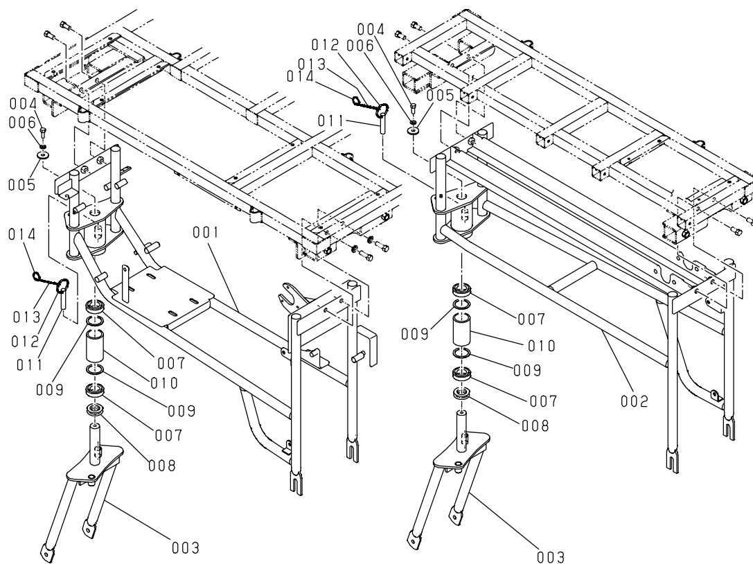
KYU-S-3 野菜運搬車
