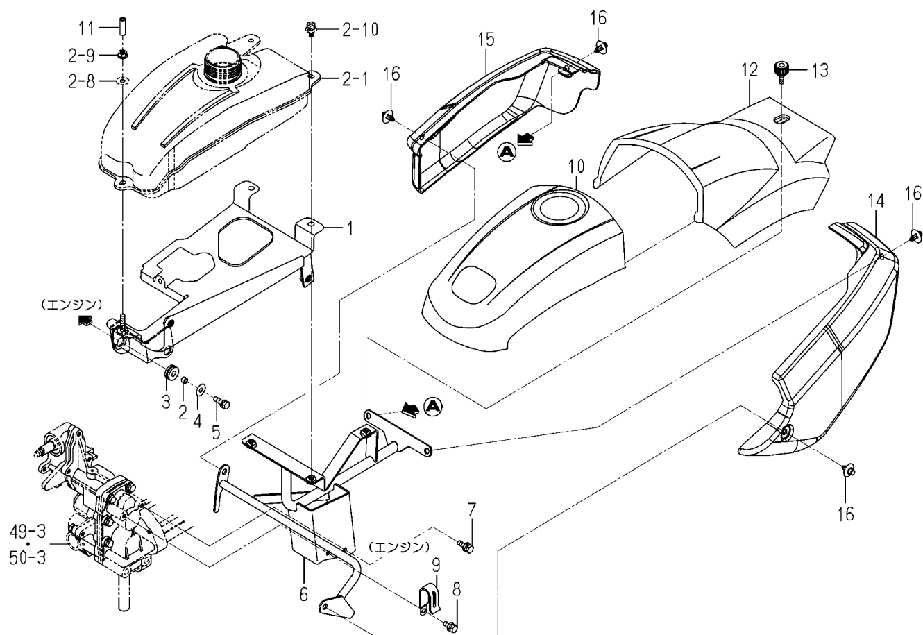
FIG. 63 フード関係
