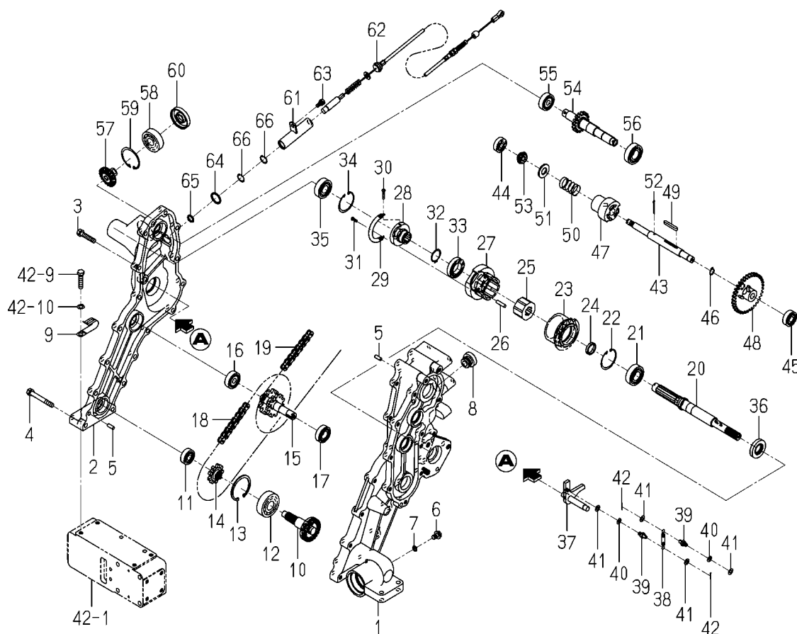
FIG. 77 フレーム(メイン)関係(X型)
