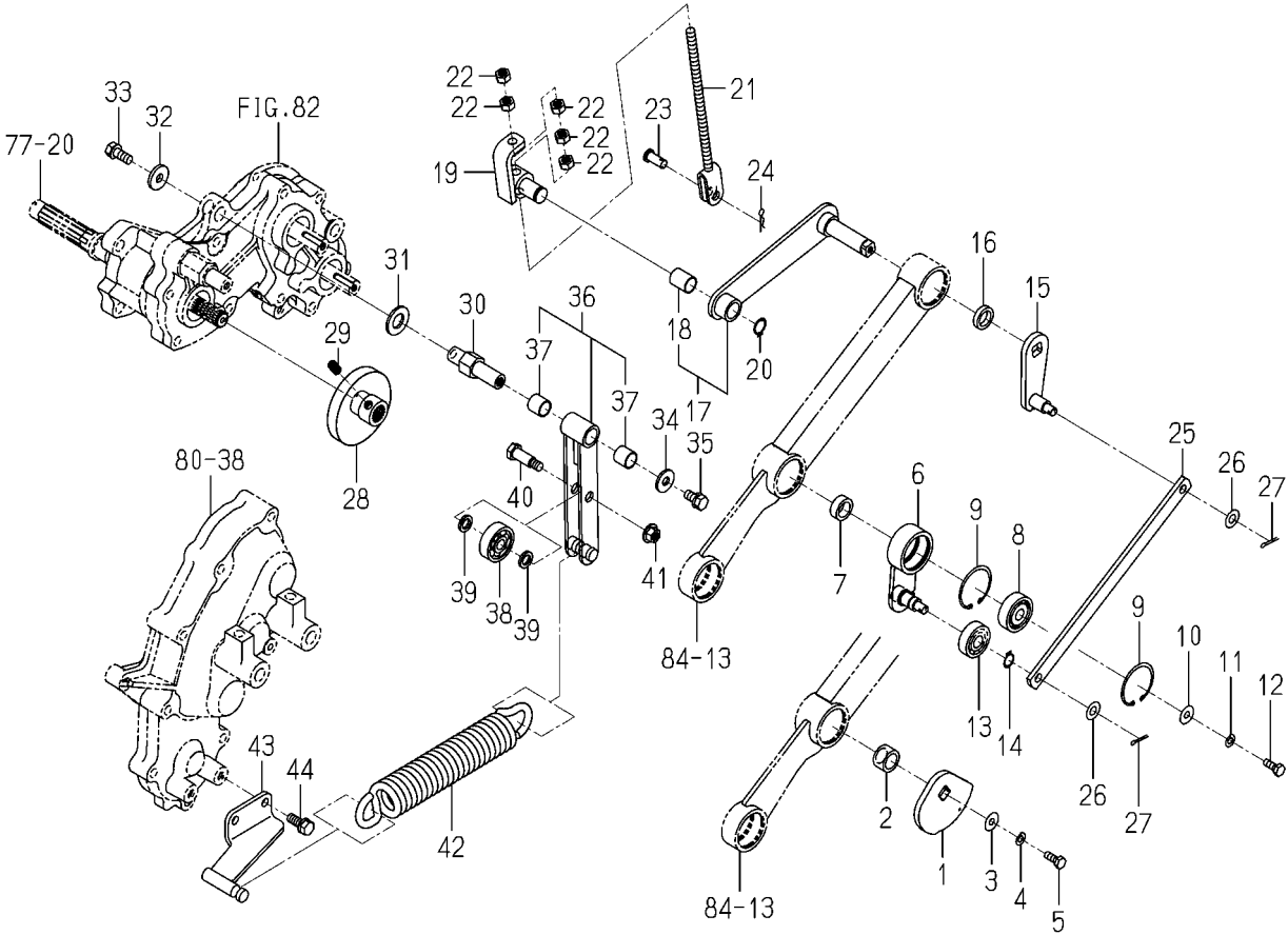
FIG. 86 カム(カイヘイ), カム(ブレーキ)関係(90JLLX型)
