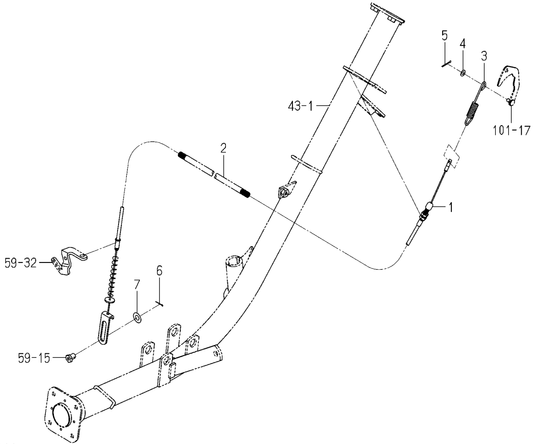
FIG.109 ケーブル(ユアツ)関係
