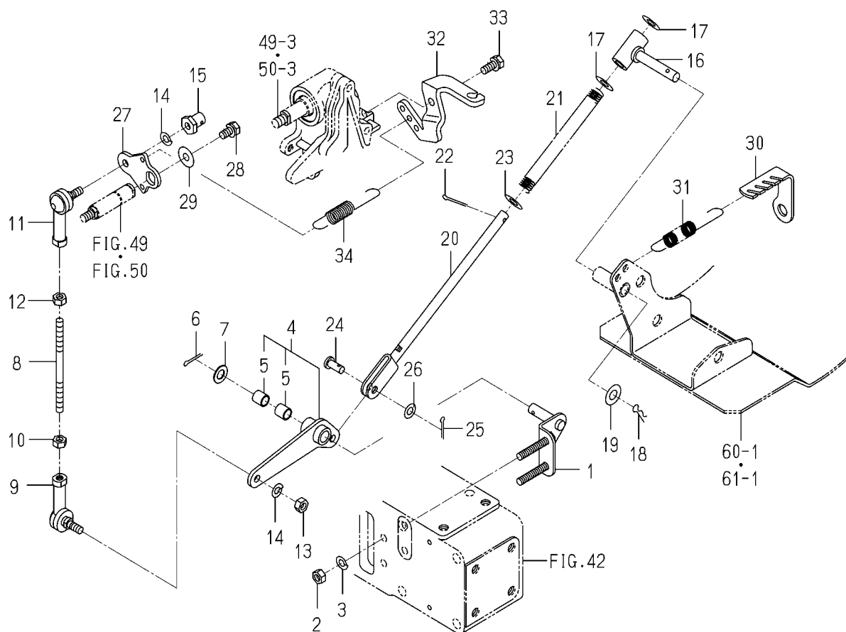
FIG. 59 ロツド(センサ／メイン)関係
