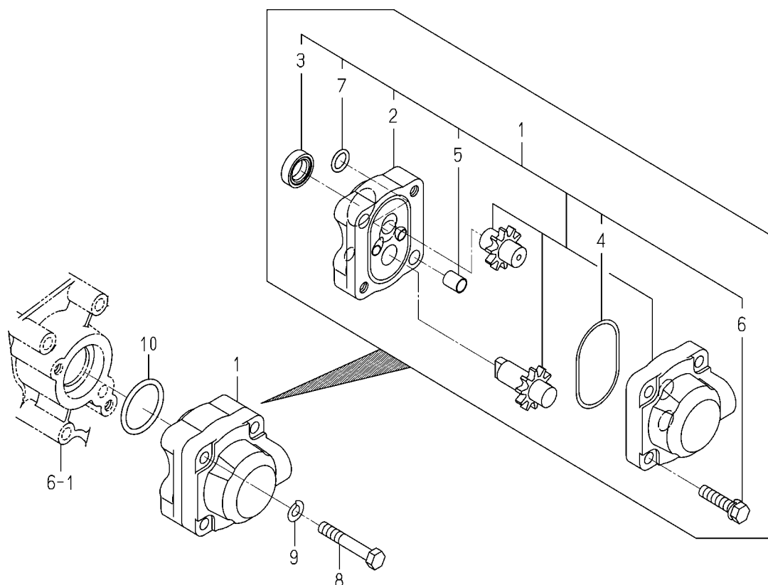
FIG. 48 ポンプ(ギヤー)関係
