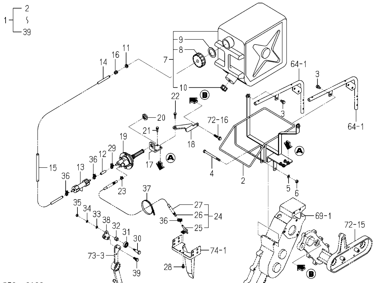
FIG.140 カンスイSET(X型除く)(オプション)
