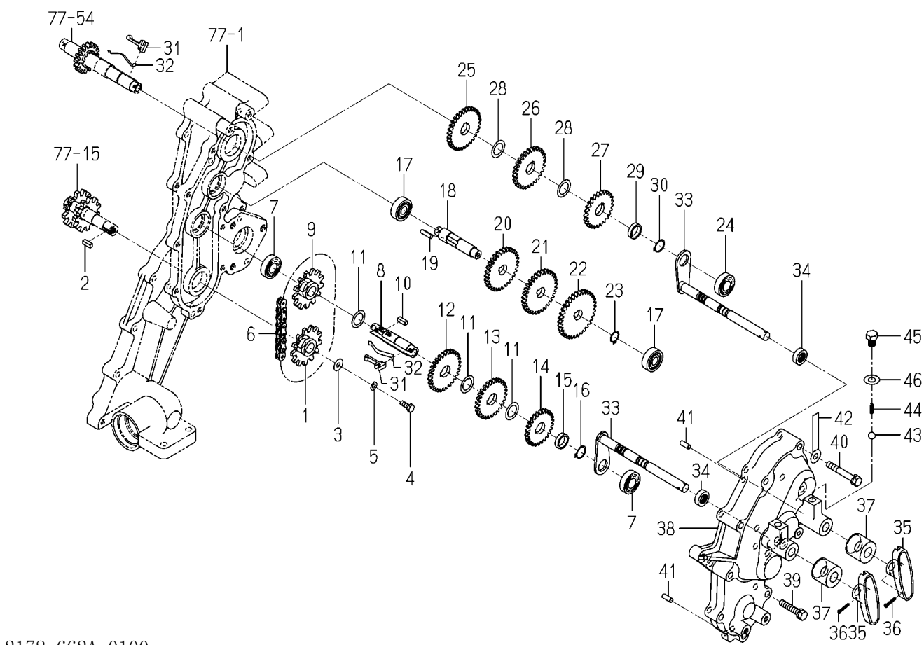
FIG. 80 ギヤー(カブマ)関係(90JLLX型)
