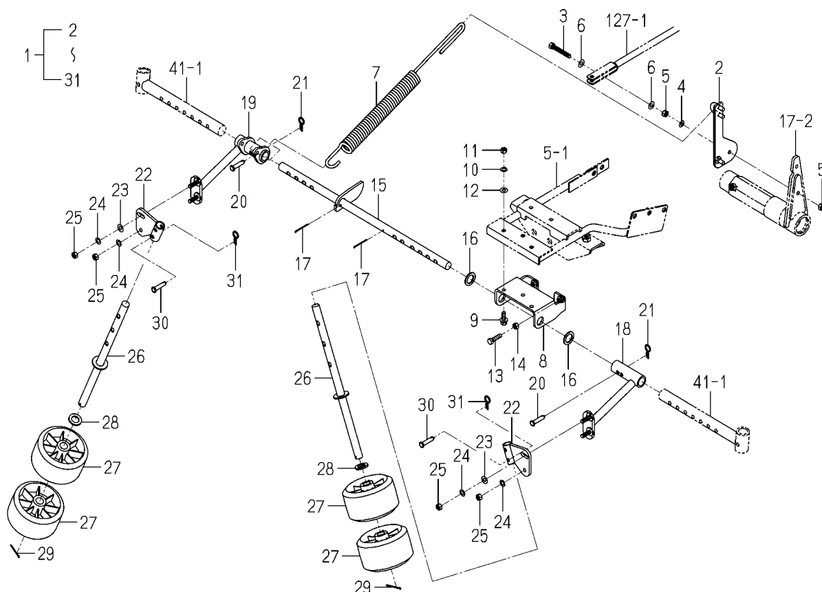
FIG.138 ガイドローラ(90J/X)SET (90JLLX型)(オプション)
