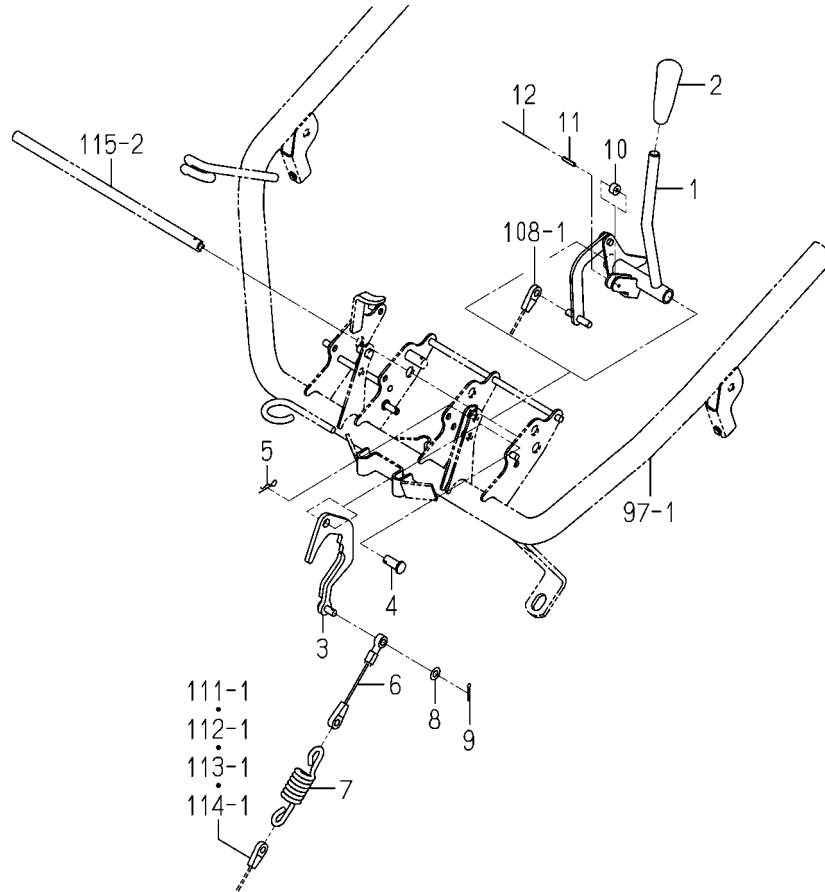
FIG.105 レバー(メイン)関係
