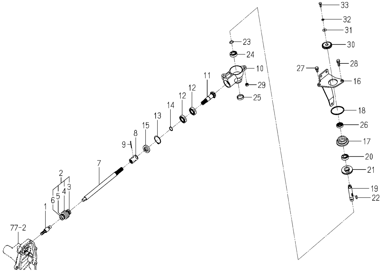
FIG. 89 ドライブ(テーブル)関係(X型)
