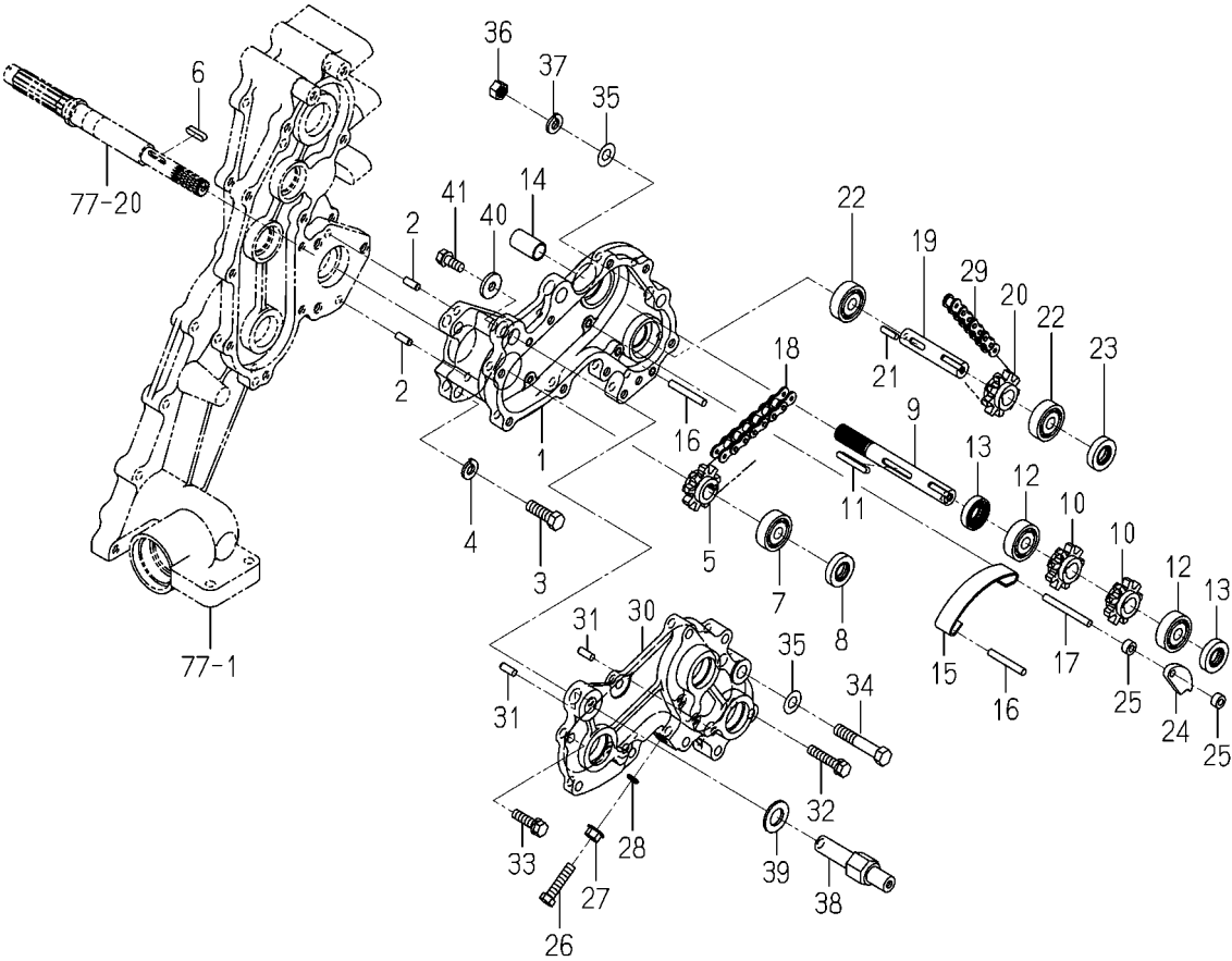
FIG. 82 ケース(クランク)関係(90JLLX型)
