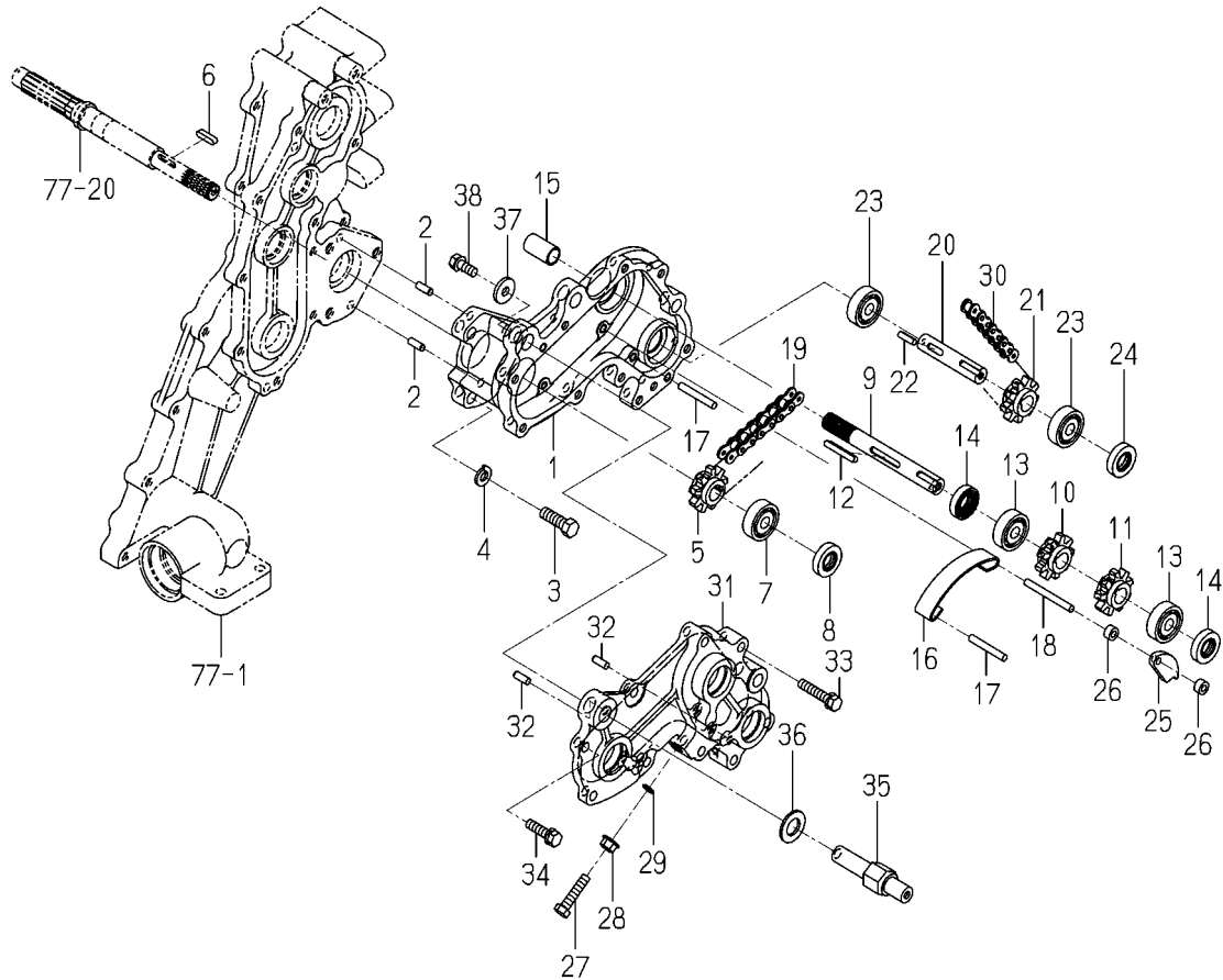
FIG. 81 ケース(クランク)関係(Jを除くX型)
