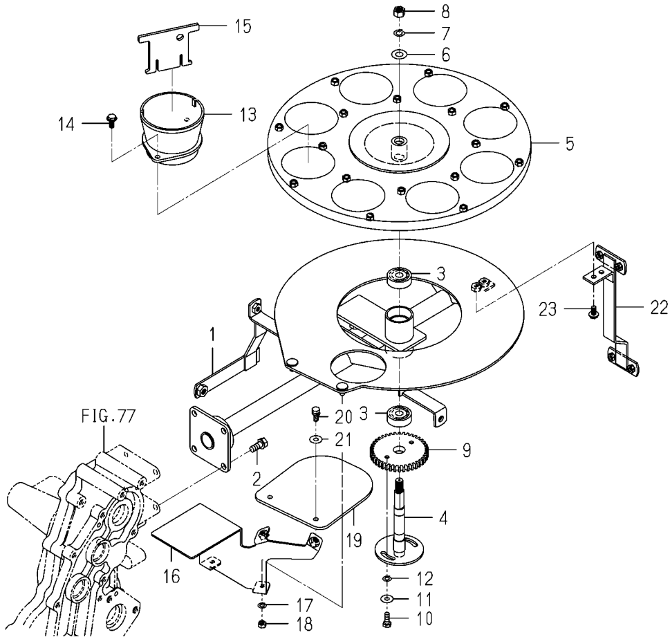
FIG. 99 テーブル関係(90JLLX型)
