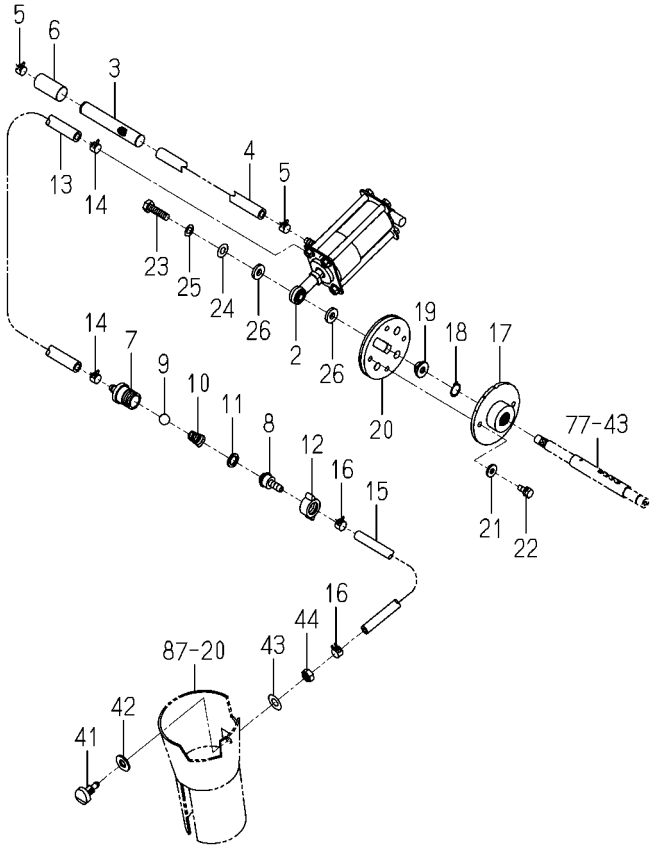
FIG.142 カンスイソウチ(100／120X)SET(図1/2) (120WLLX型)(オプション)
