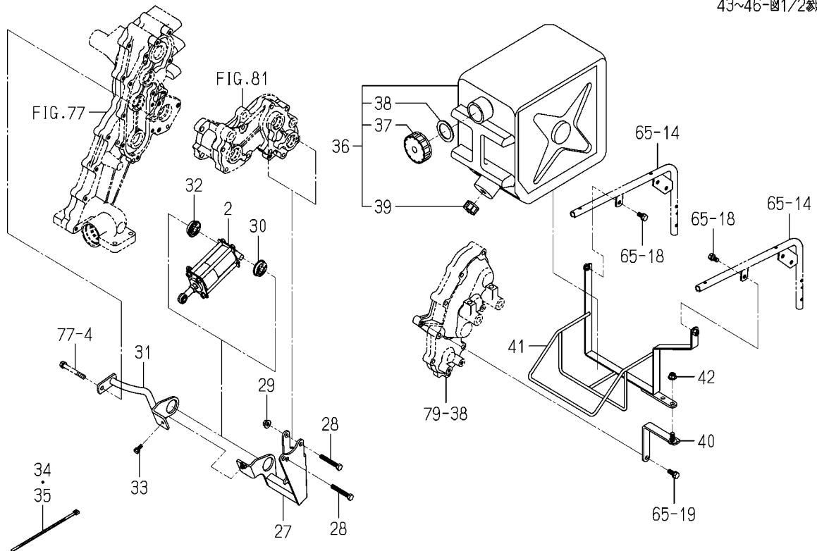
FIG.141 カンスイソウチ(100／60X)SET(図2/2) (Xを除く60型)(オプション)
