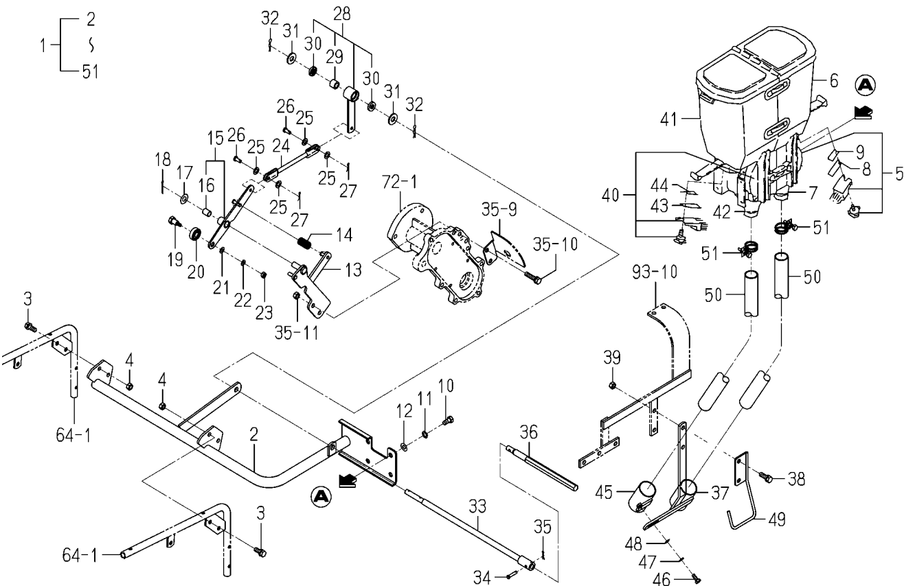
FIG.145 ヤクザイサンプキ(2レン)SET(X型除く)(オプション)
