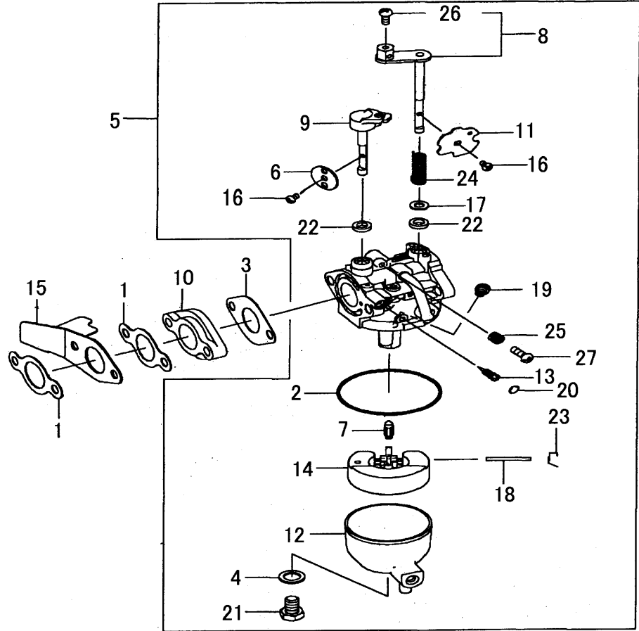
FIG. 8 キャブレタ
