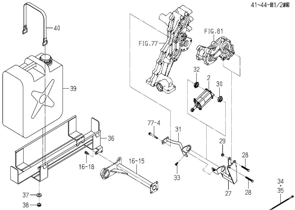
FIG.142 カンスイソウチ(100/120X)SET(図2/2) (120WLLX型)(オプション)
