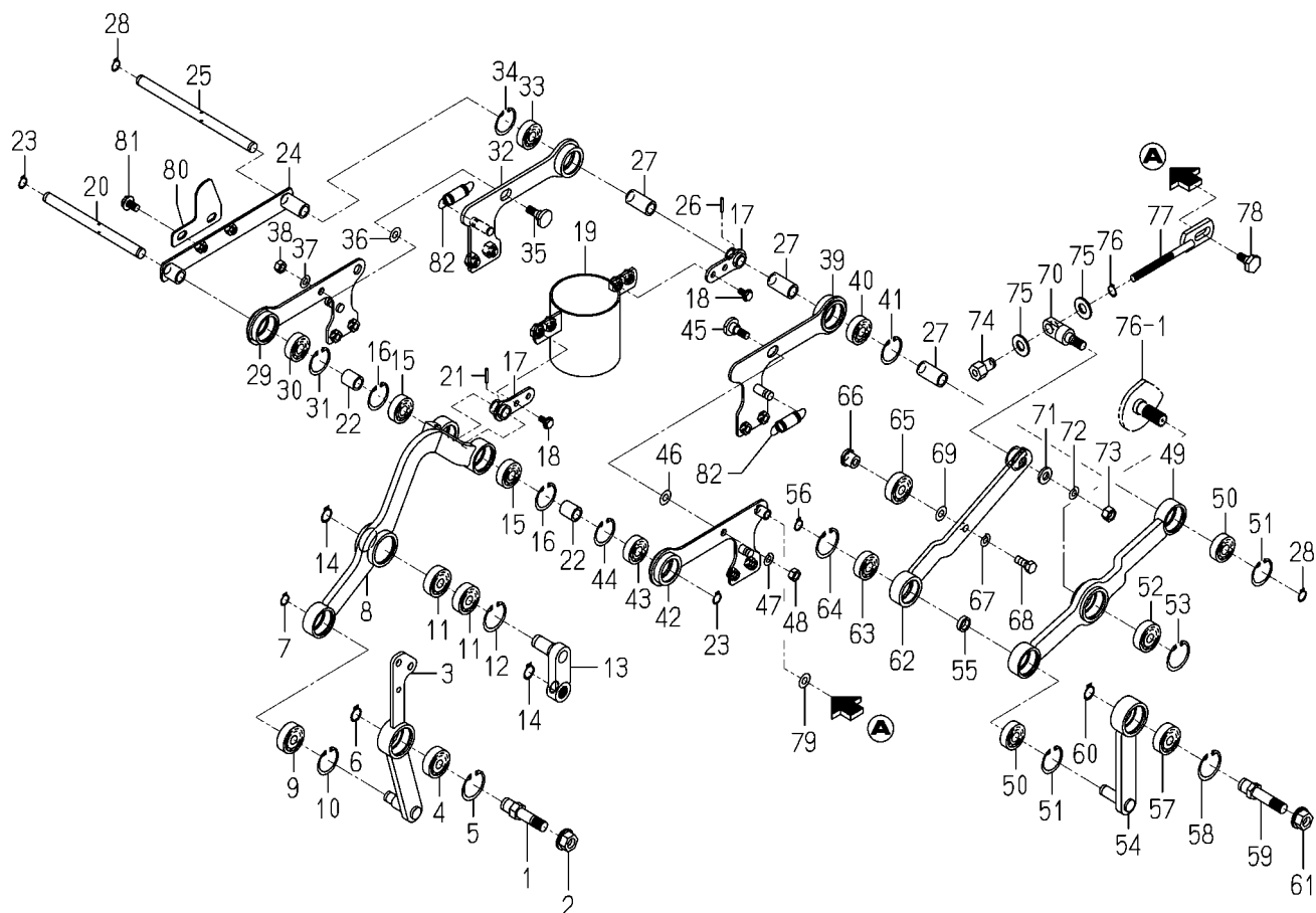
FIG. 73 リンク関係(X型除く)
