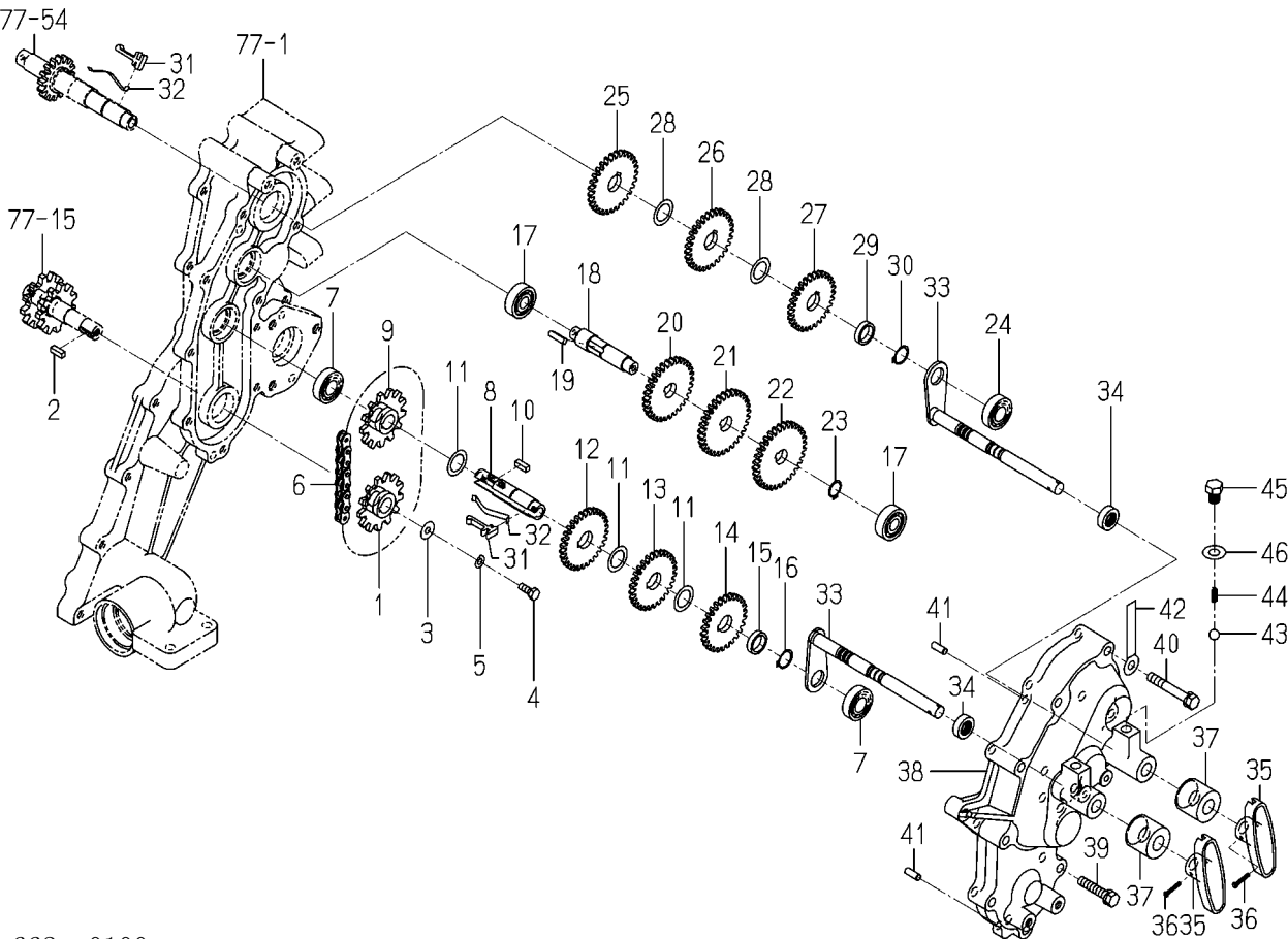
FIG. 79 ギヤー(カブマ)関係(Jを除くX型)
