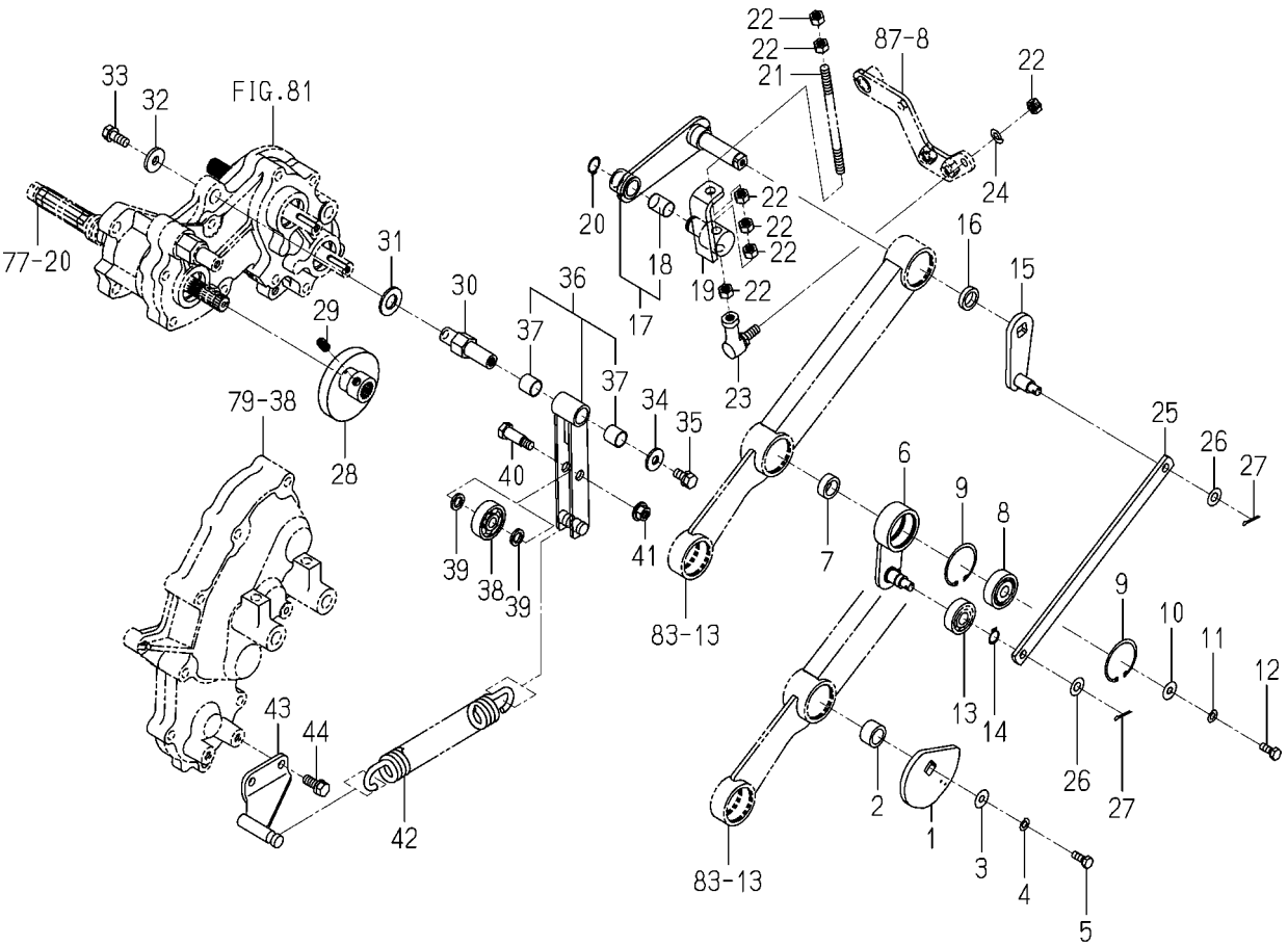
FIG. 85 カム(カイヘイ), カム(ブレーキ)関係(Jを除くX型)
