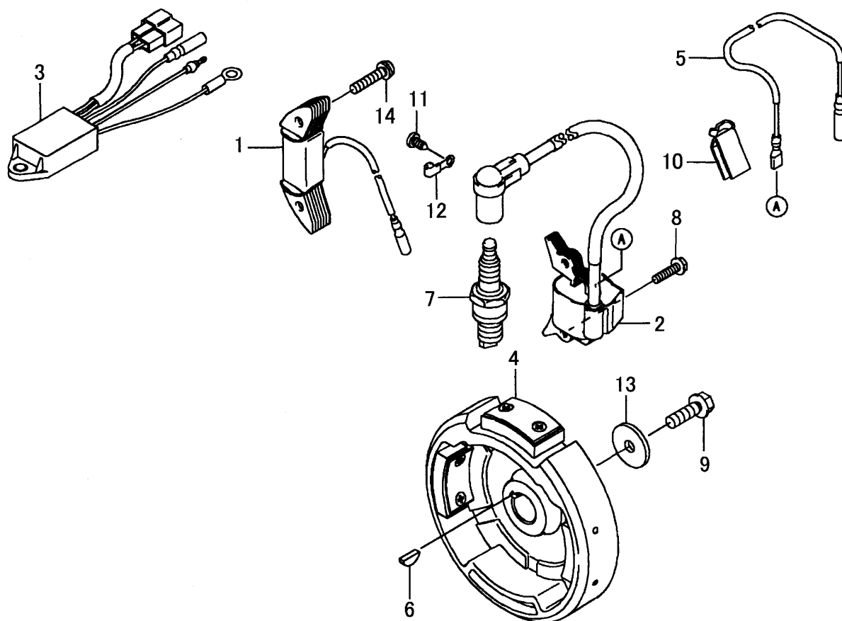
FIG. 6 デンソウヒン
