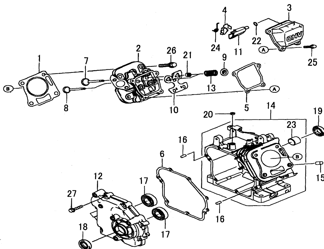
FIG. 1 シリンダ／クランクケース
