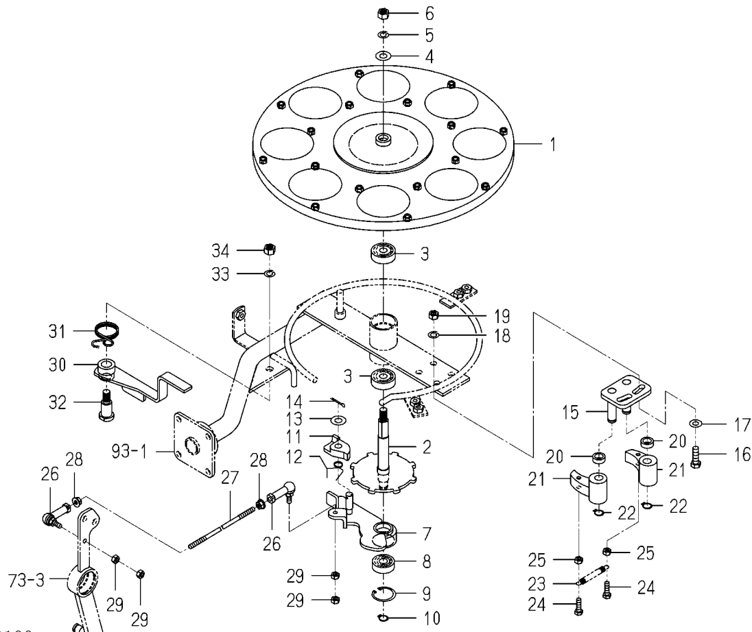
FIG. 94 ターン(テーブル)関係(X型除く)
