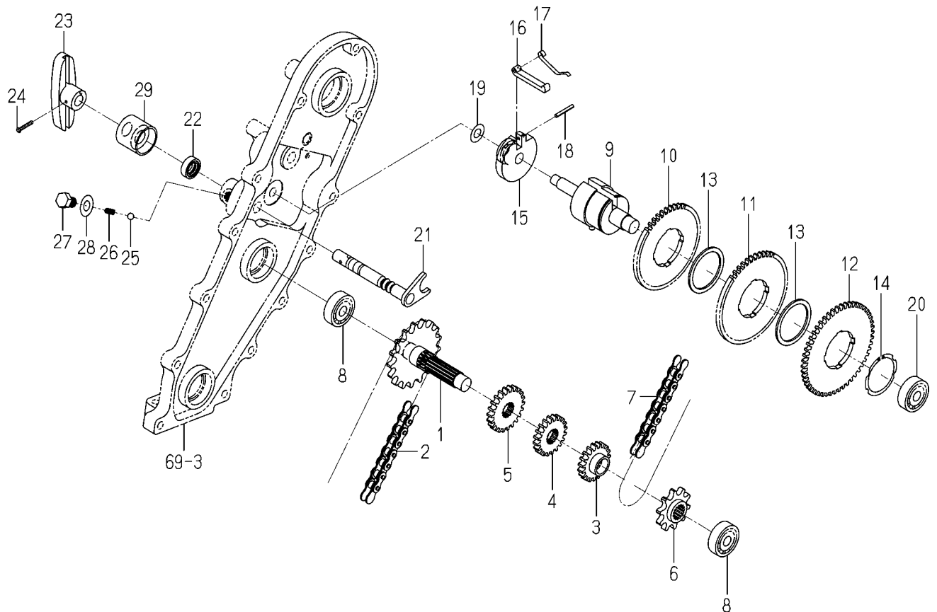
FIG. 71 ギヤー(カブマ)関係(X型除く)
