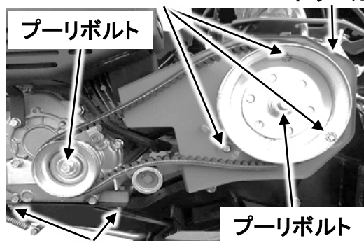
エンジン固定ボルト(4本)
