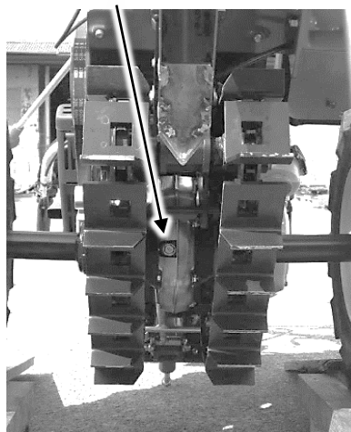
排油プラグ
