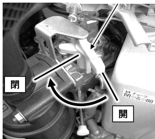
チョークレバー
