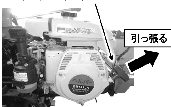
リコイルスタータハンドル
