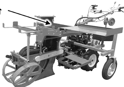
苗搬送台
