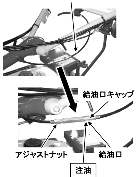
ハンドル上下調節ケーブル
