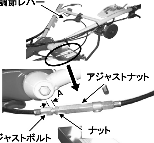
ハンドル上下 調節レバー
