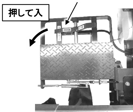
主クラッチペダル
