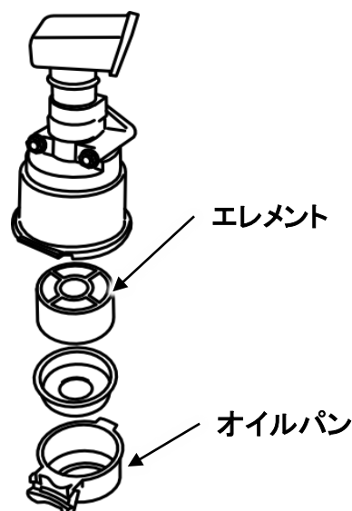
エアクリーナー分解図
