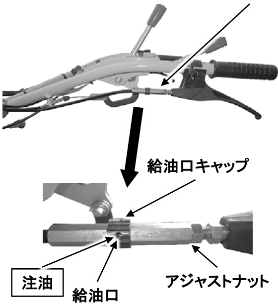
サイドクラッチ(左)ケーブル
