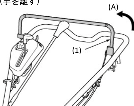
(1) 主クラッチレバー
