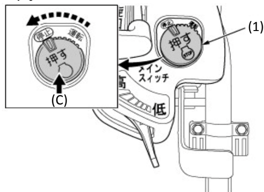
(1) メインスイッチ (C) 押す
