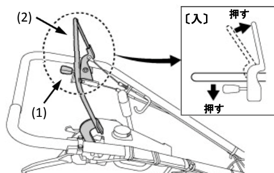
(1) 駐車ブレーキロックレバー (2) 主クラッチレバー
