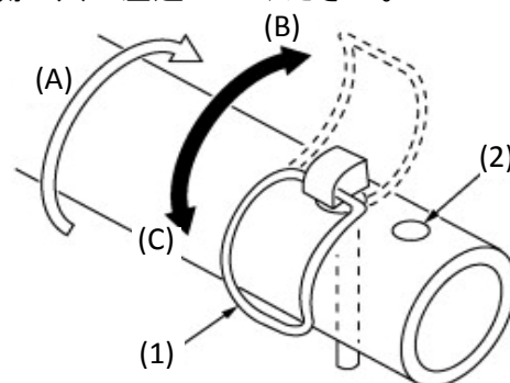
(1) セットピン (2) 白色合いマーク (A) 爪軸回転方向 (B) 解除 (C) 固定
