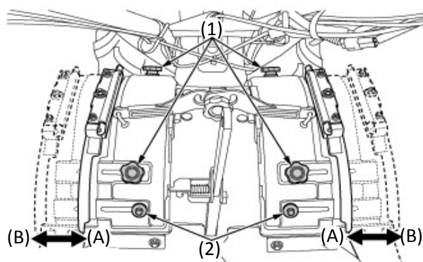
(1) ノブナット (2) 回り止めナット (A) 狭める (B) 広げる
