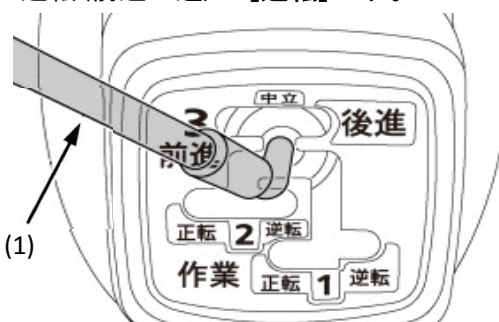
(1) 主変速レバー
