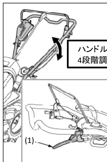
(1) ハンドル上下調節レバー
