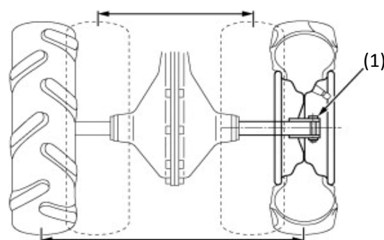
(1) 車輪取付ピン
