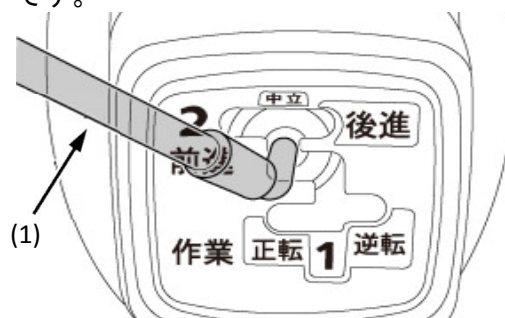
(1) 主変速レバー
