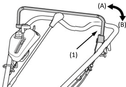
(1) 主クラッチレバー (A) [切] (B) [入]
