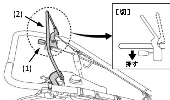
(1) 駐車ブレーキロックレバー (2) 主クラッチレバー
