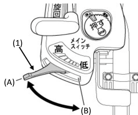
(1) スロットルレバー (A) 【高】 (B) 【低】
