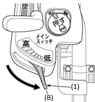
(1) スロットルレバー (B) [低]
