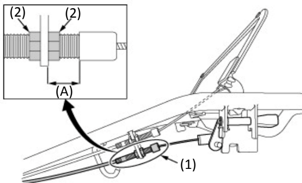
(1) 駐車ブレーキ調節金具 (A) 幅を調節 (2) ロックナット
